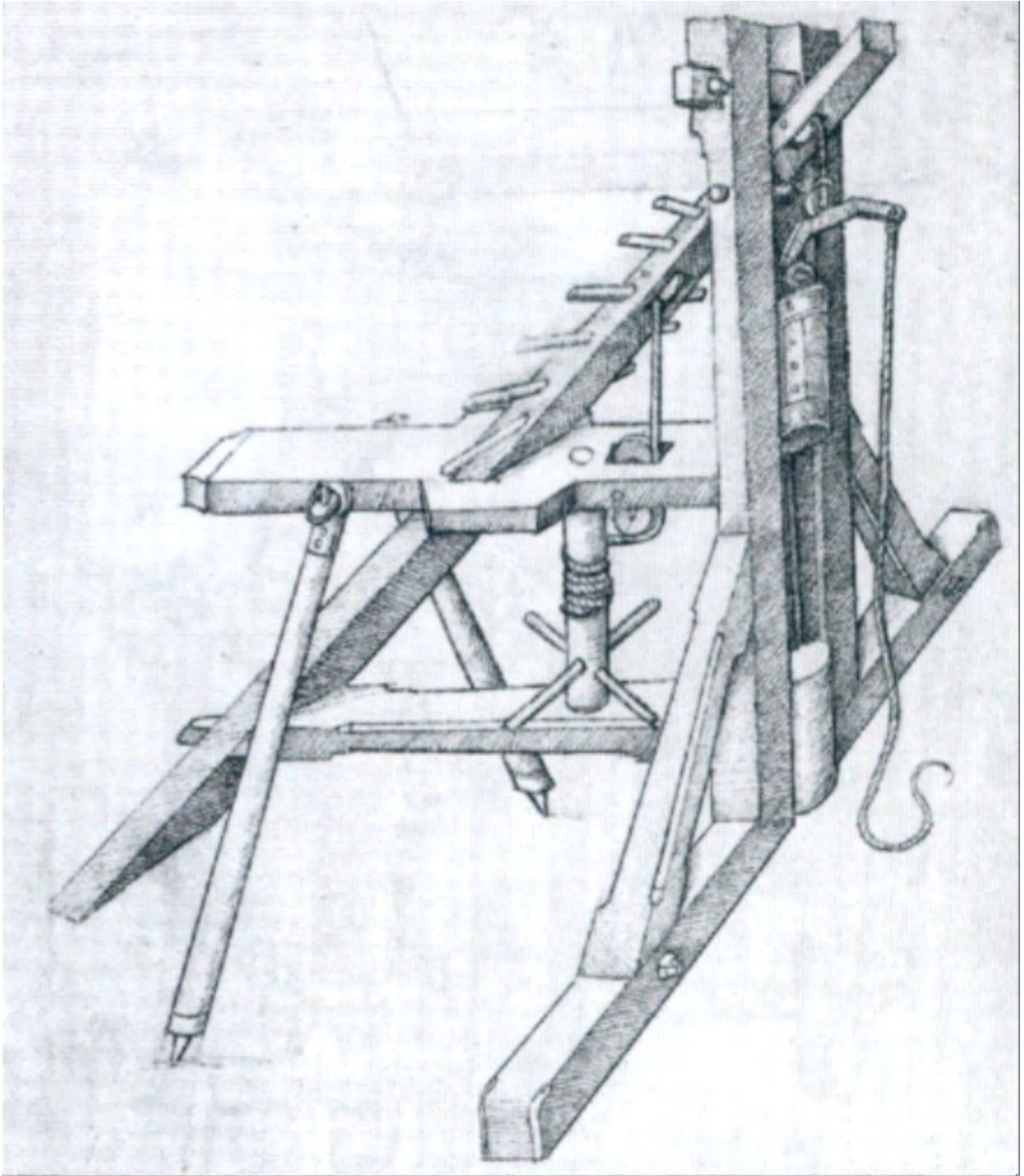
RUČNÍ BERANIDLO PRO ZARÁŽENÍ PILOTŮ 1480
